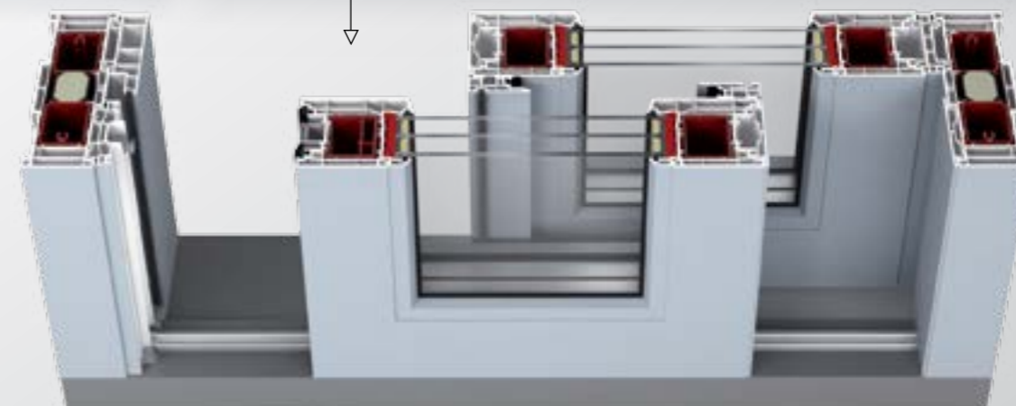
Drzwi HST 85 mm, schemat A, okleina AP 61
